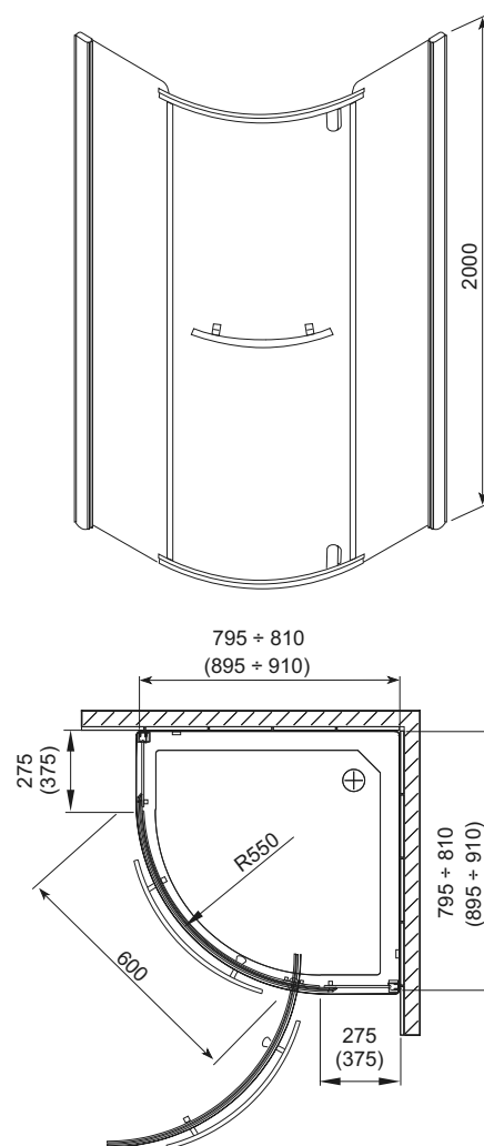
PUENTA WIND - кабіна ліва
